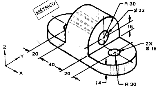
Figura 6-6-F Bloque en almohada.
