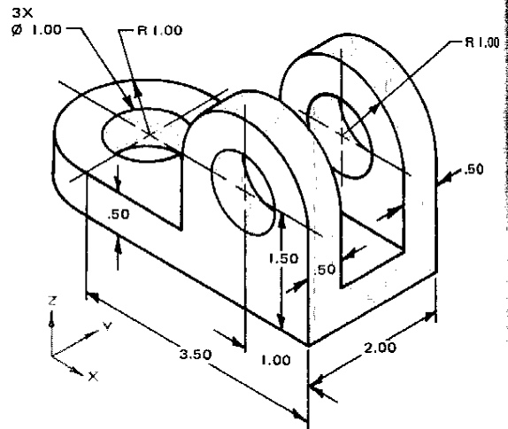
Figura 6-6-L Brazo oscilante.
