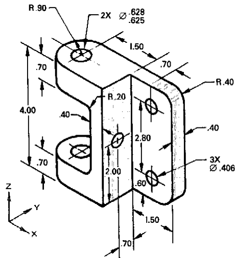
Figura 6-6-H Sostén de bisagra.
